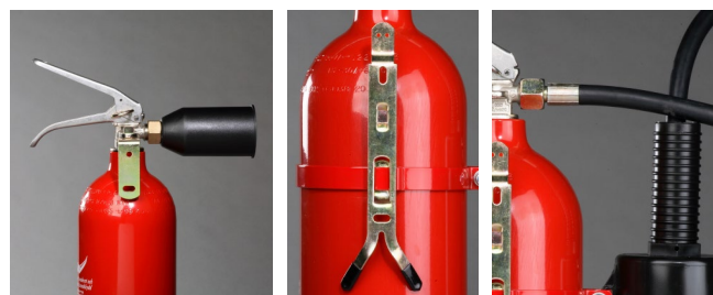
2 kg släckaren har snörör monterat på ventilen och en krok för väggmontage.
